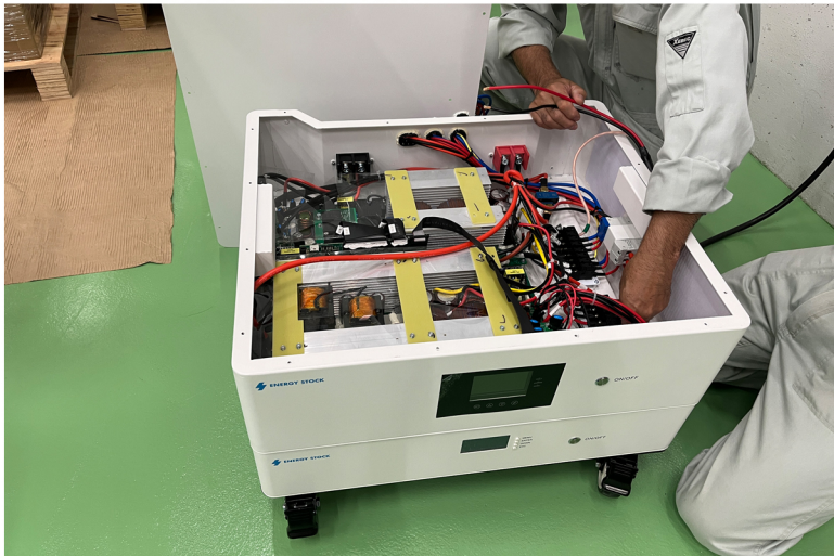
PV（ソーラーパネル配線接続）外部電源接続
